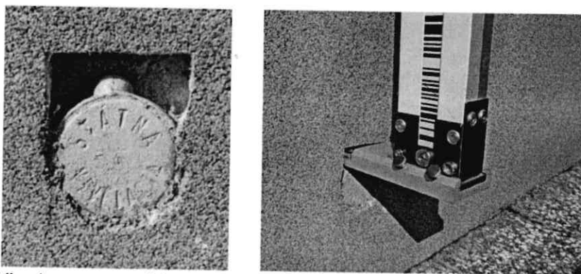
Obr. 2 Vhodne upravená fasáda okolo nivelačného bodu pri geodetickom meraní
