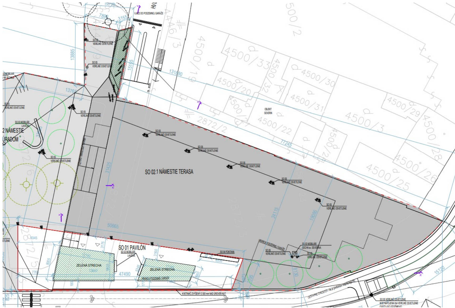
Koordináčna situácia
